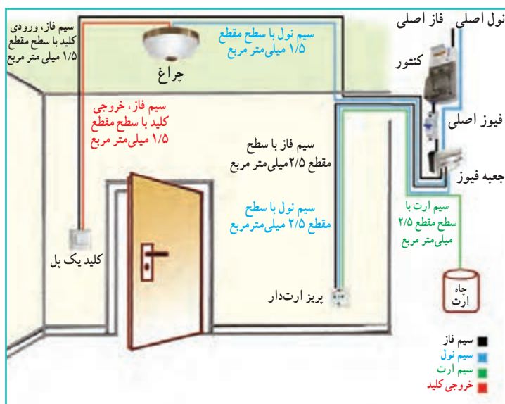
الف - سیم کشی داخل ساختمان، کلید یک پل با یک لامپ و یک پریر
